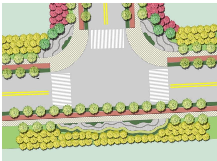
图 2.2-8 路口平面图
