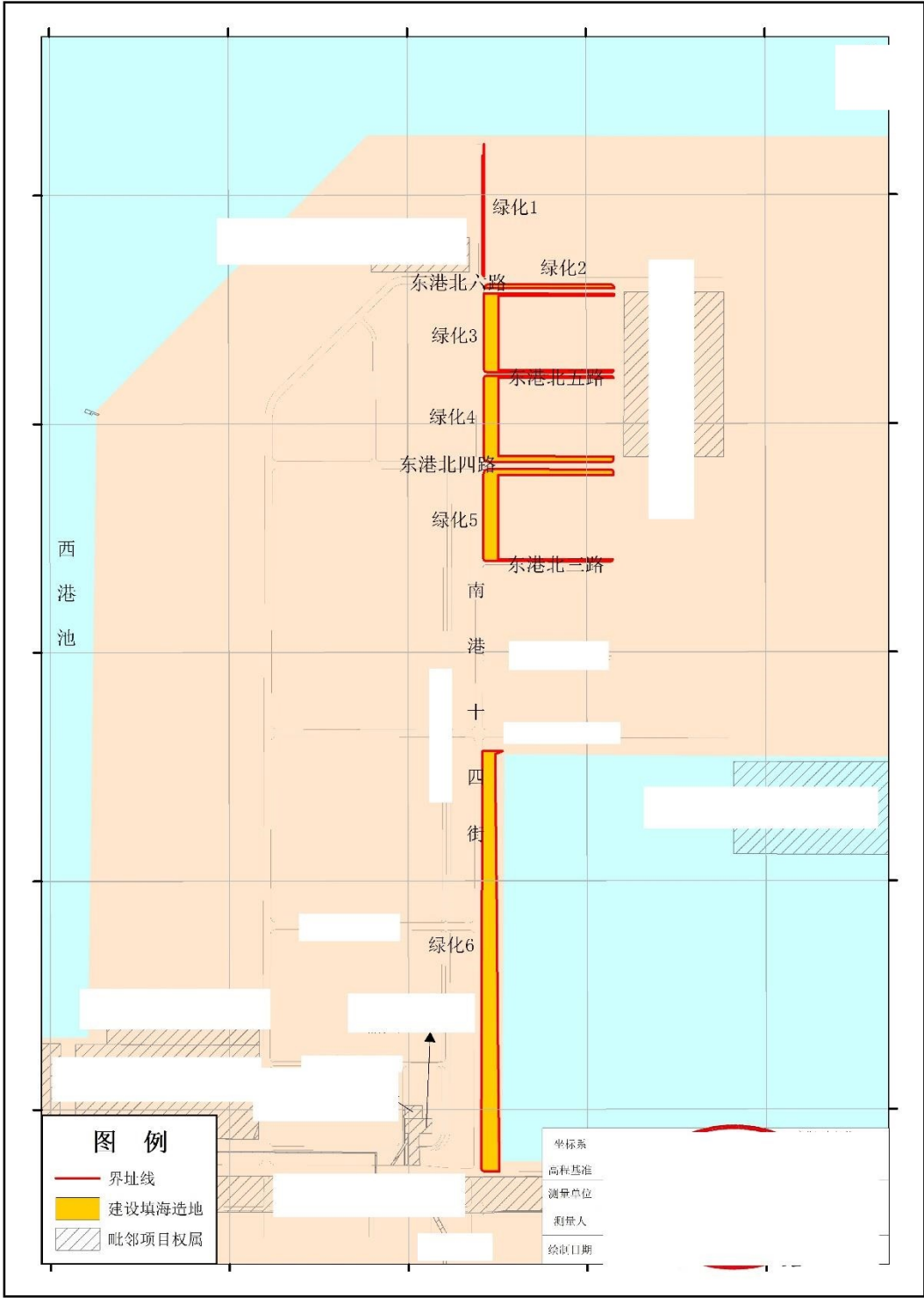
图 7.3-5 东区绿化工程宗海平面布置图 (***)
