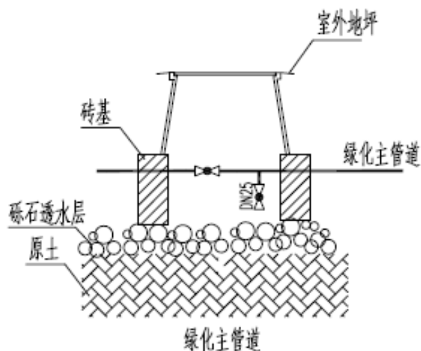
图 2.3-5 给水阀门井安装示意图
