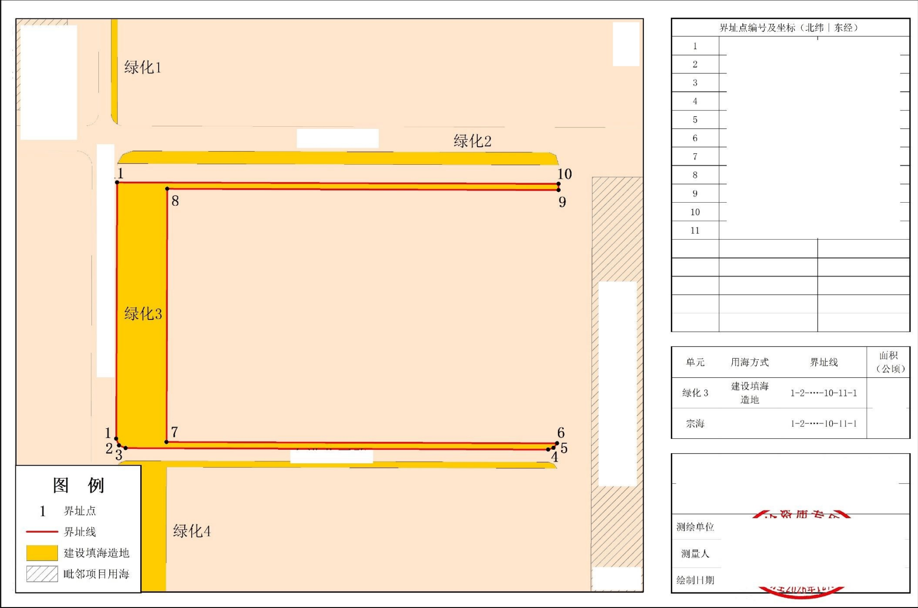
图 7.3-11 东区绿化工程 3 宗海界址图 (***)
