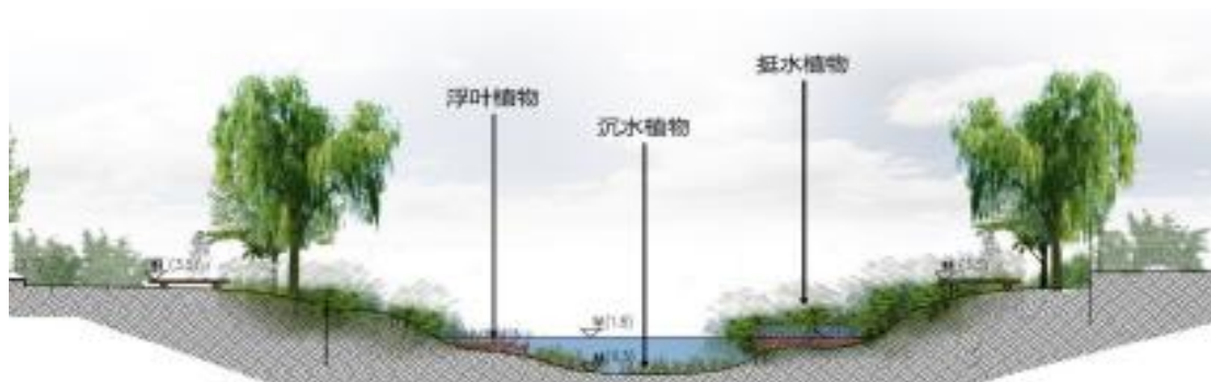
图 2.2-7 设计断面图
