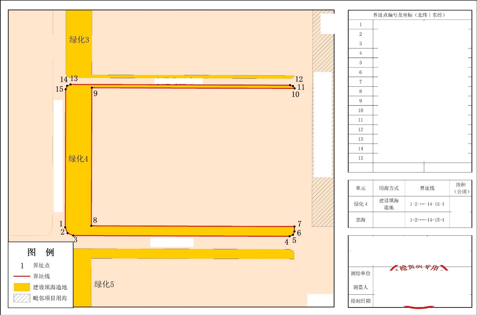
图 7.3-13 东区绿化工程 4 宗海界址图 (***)
