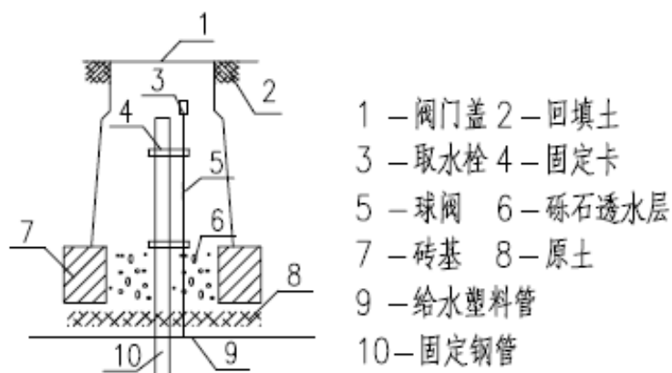
图 2.3-5 给水阀门井安装示意图
