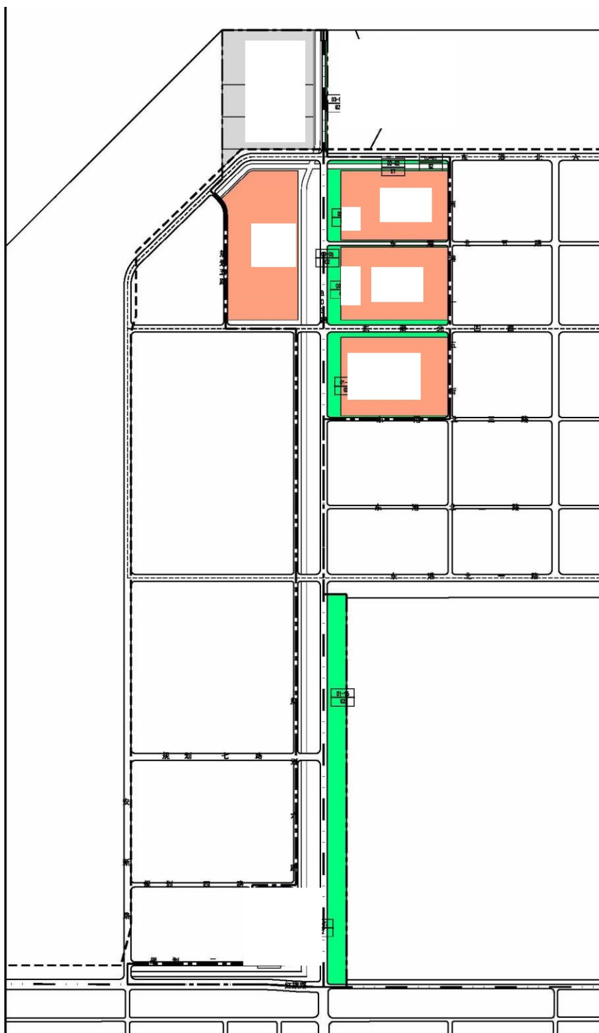
图 7.3-1 平面布置图
