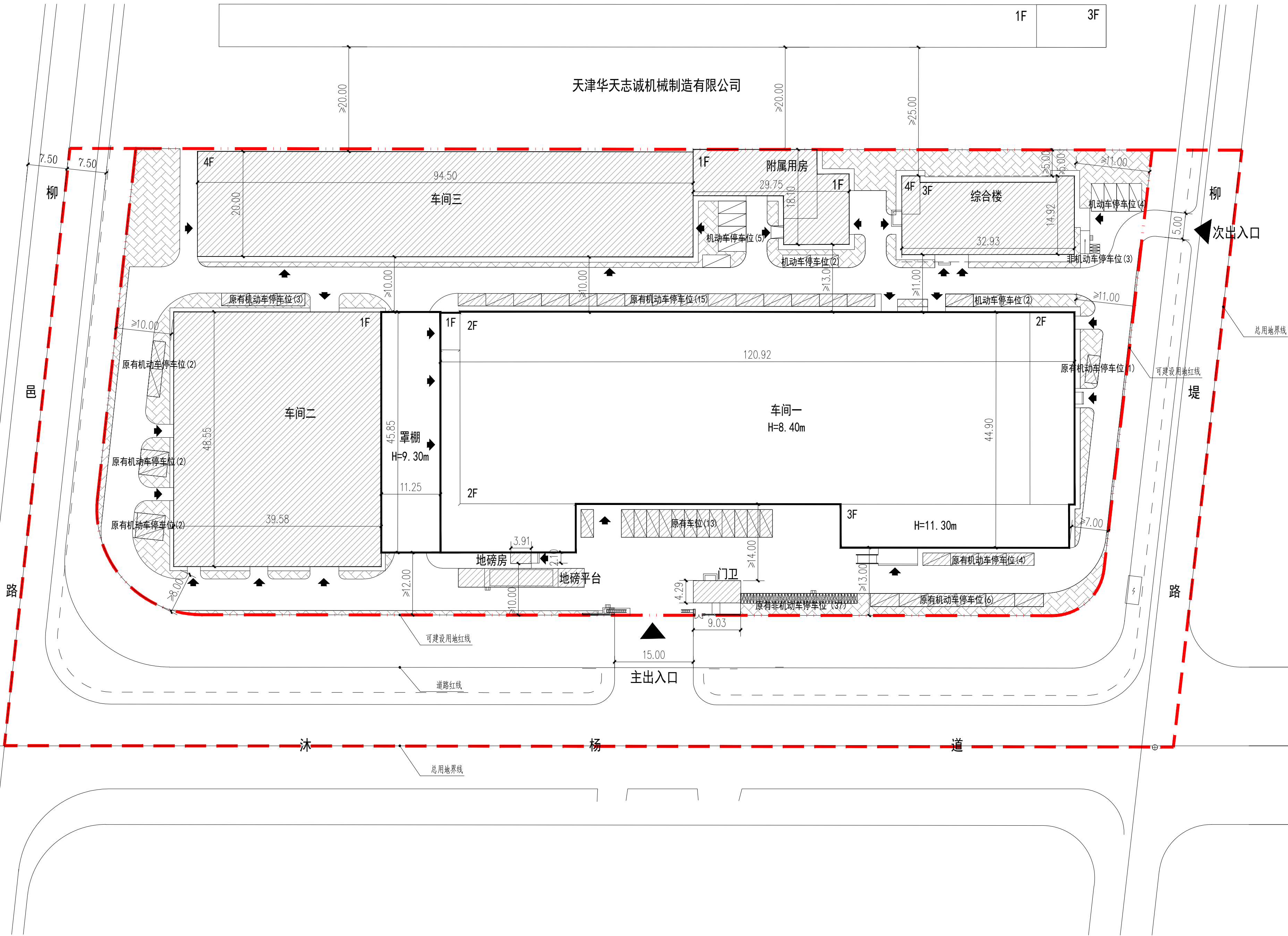
总平面图 1:500
