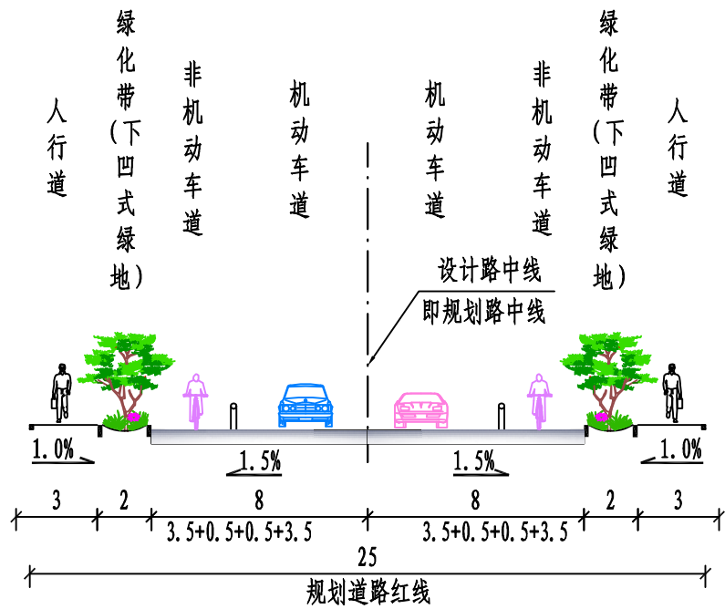
标准横断面设计图
