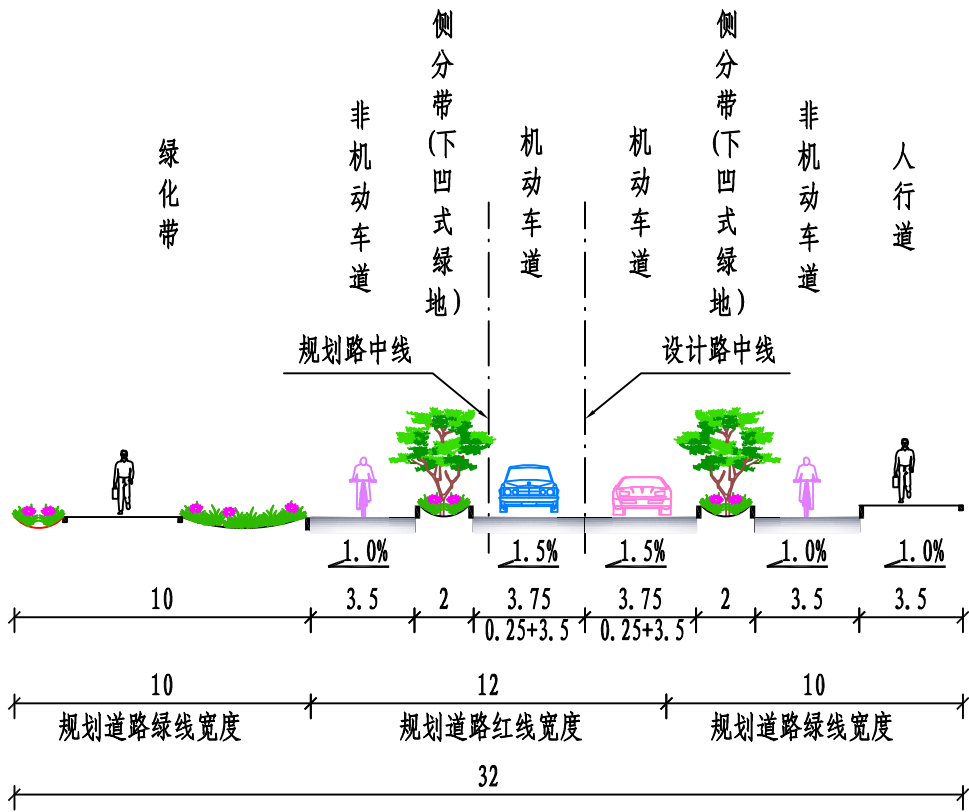
标准横断面设计图
