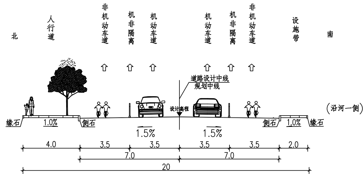
道路标准横断面
