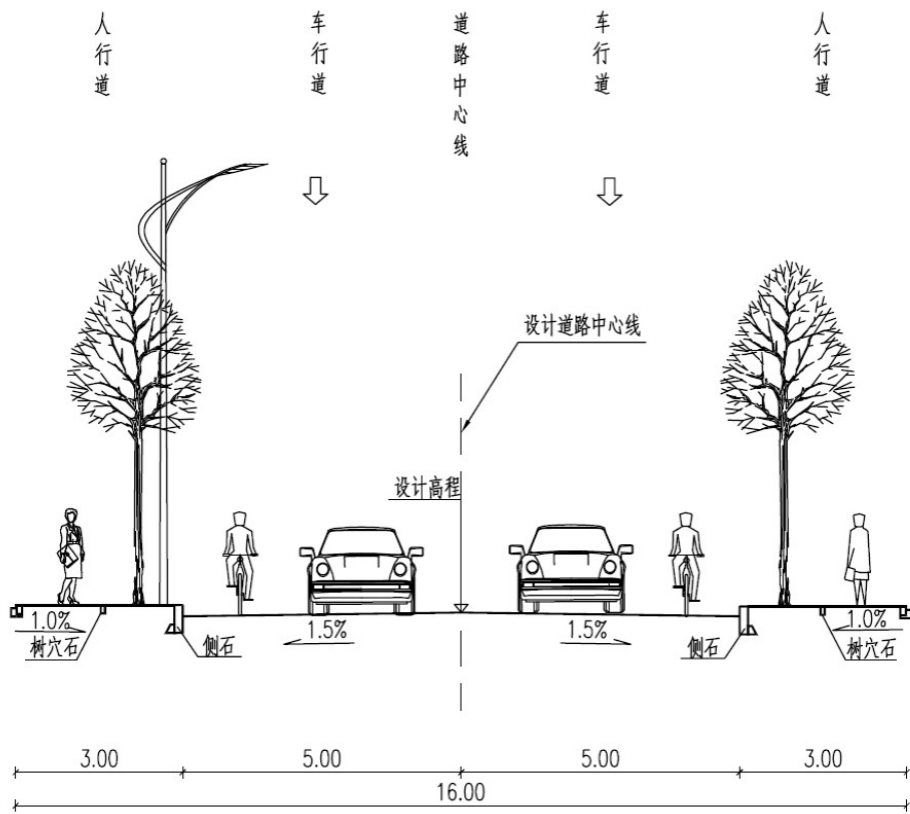
道路标准横断面图
