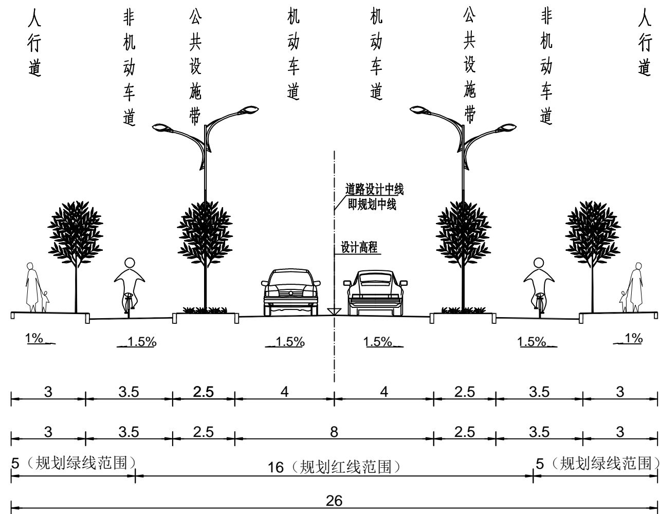
标准横断面设计图
