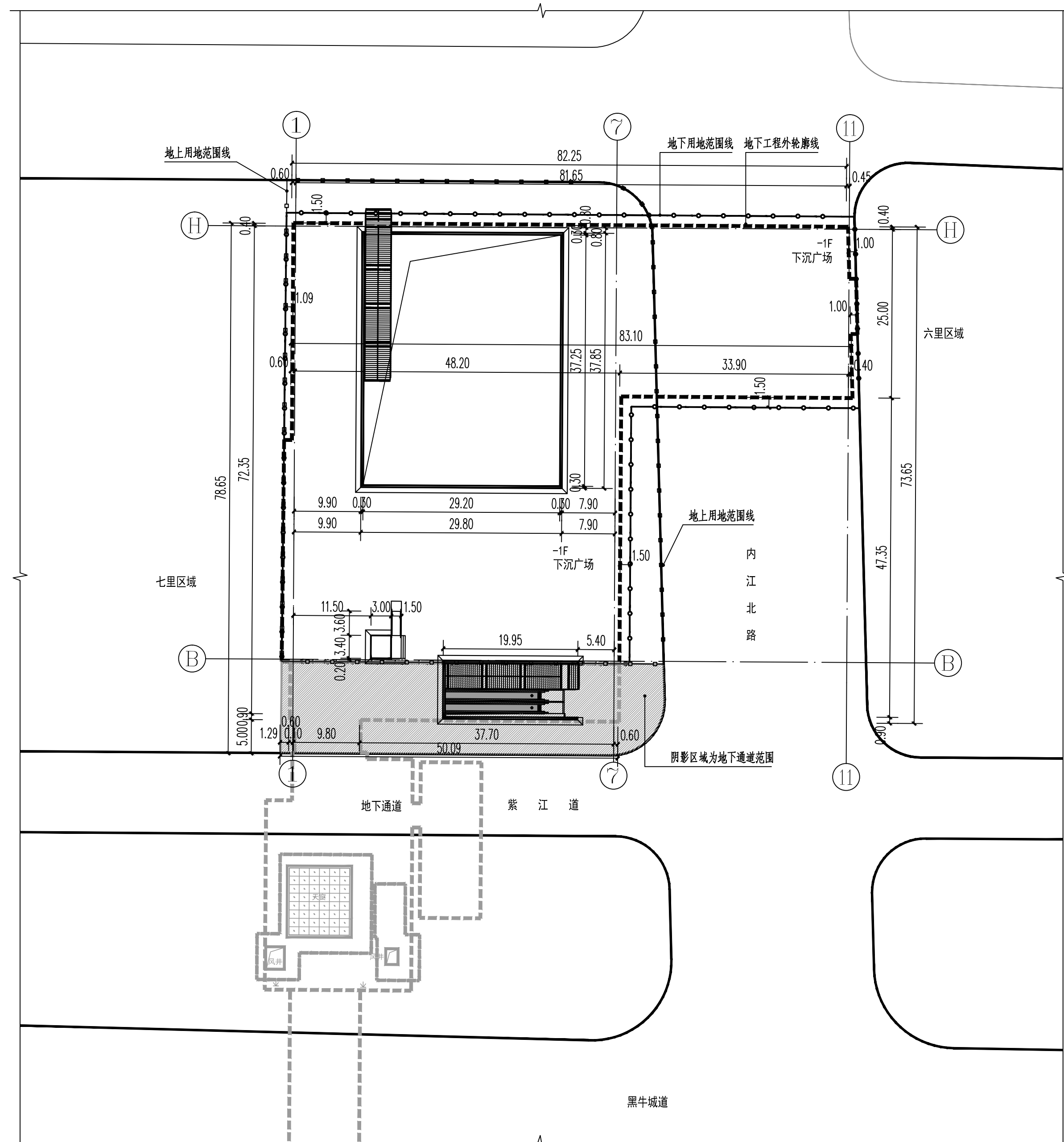
总平面图 1:500
